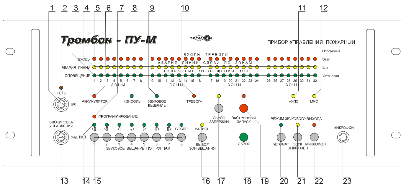
Рис. 1. Внешний вид ППУ «Тромбон – ПУ-М» и расположение органов управления и индикации.
