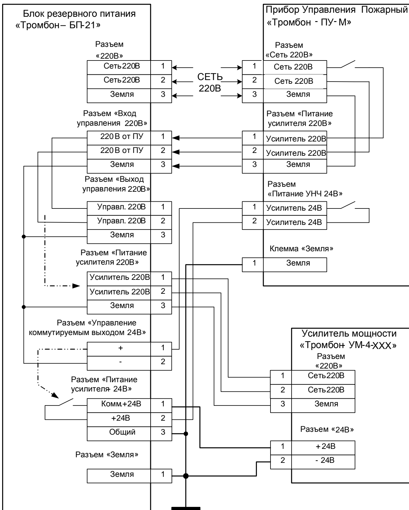
Схема управления питанием одного усилителя мощности с одним блоком резервного питания.
