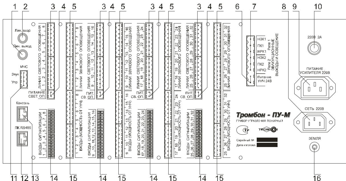
Рис. 2. Прибор управления пожарный, вид со стороны задней панели.
