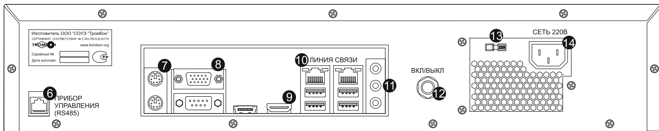
Рис. 2. Задняя панель Блок «Тромбон – БЧС».
