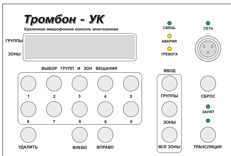
Рис. 3. Внешний вид удаленной консоли «Тромбон – УК-М».
