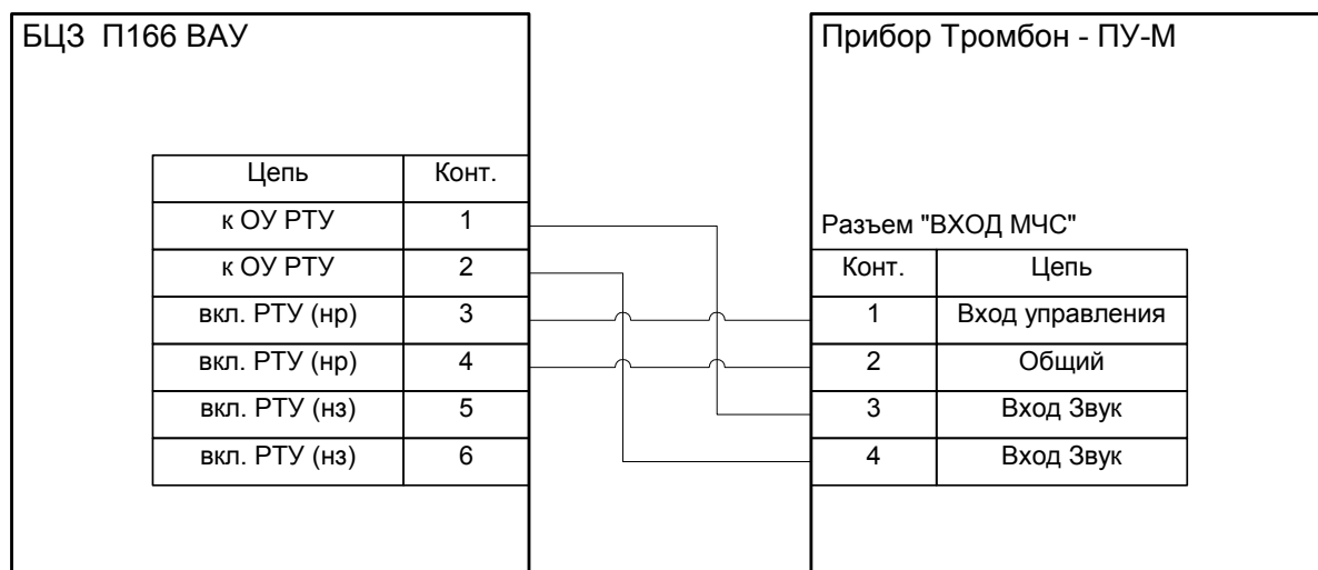
Схема подключения каналов управления и оповещения МЧС к прибору "Тромбон - ПУ-М" при использовании Блока централизованного запуска МЧС (БЦЗ) - П166 ВАУ
