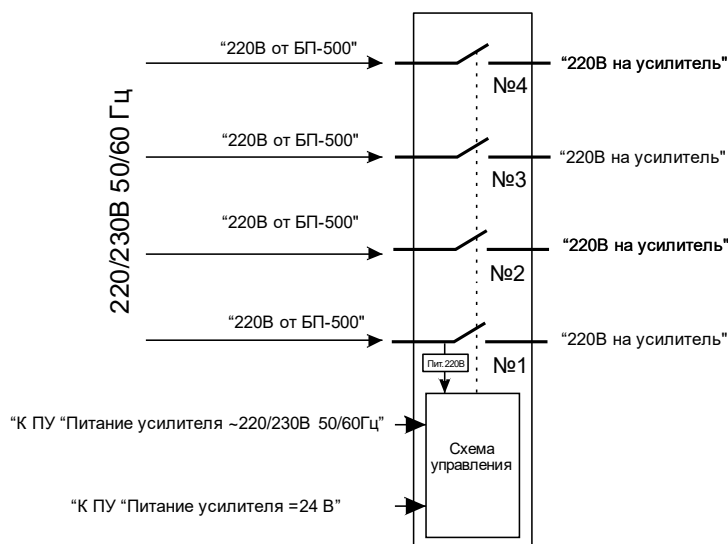
Рис. 1. Блок коммутации Тромбон – БК структурная схема
