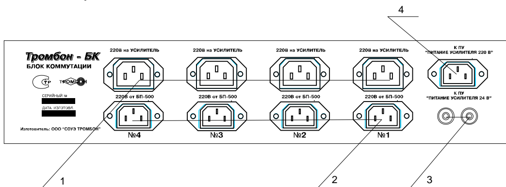
Рис. 3 Эскиз задней панели Блока
