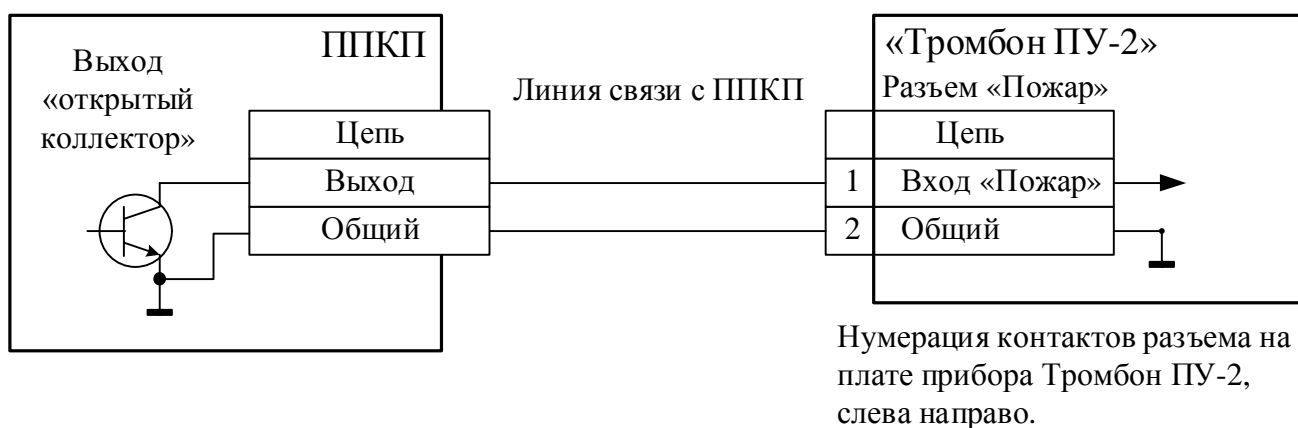
Рис. 6. Схема подключения к ППКП с выходом «Открытый коллектор» без контроля исправности линии связи.
