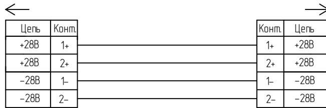
Распайка силового кабеля
