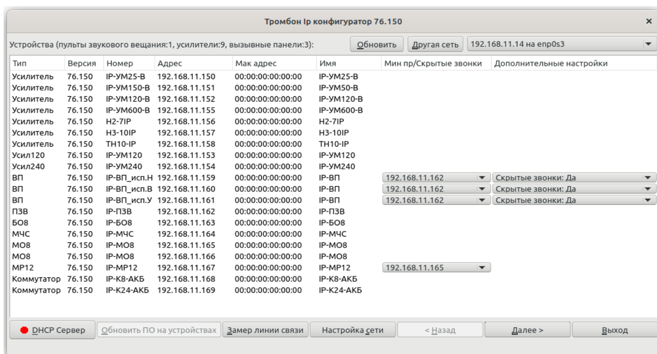
Рисунок 6 - Версия обновлена
