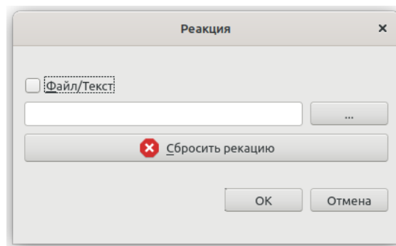
Рисунок 26 - Настройка реакции
