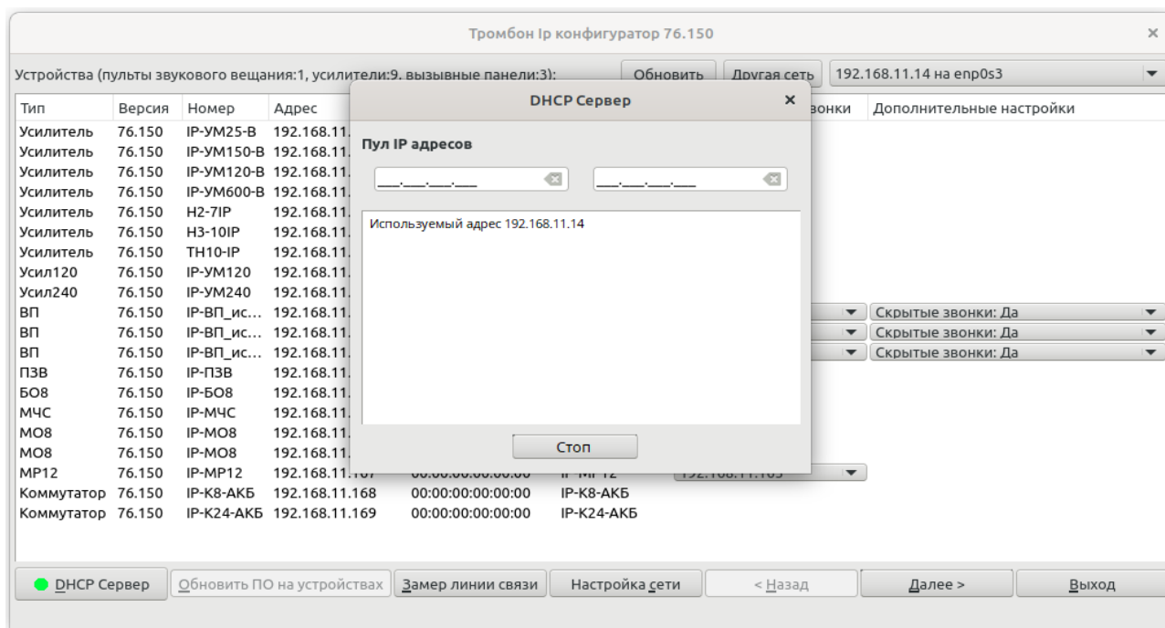
Рисунок 9 - DHCP сервер
