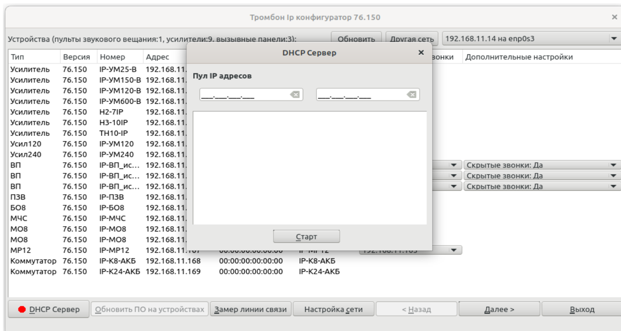
Рисунок 8 - DHCP сервер
