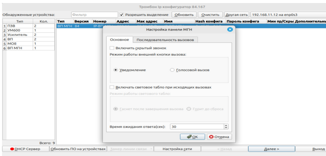
Рисунок 16 - Настройка панелей
