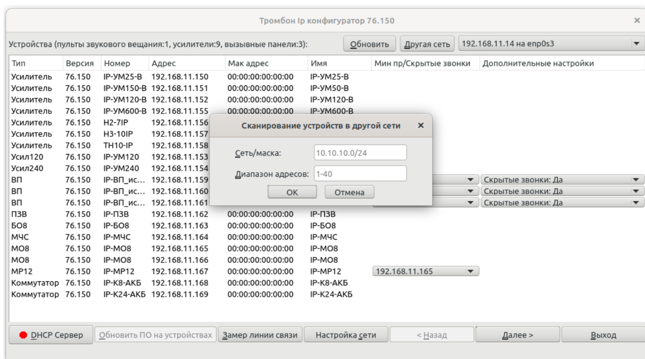
Рисунок 4 - Другая сеть
