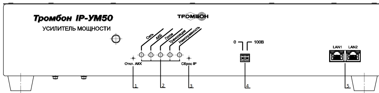
Рисунок 2 - Вид спереди
