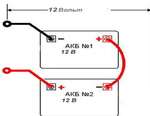
Рисунок 4 - Схема подключения аккумуляторных батарей
