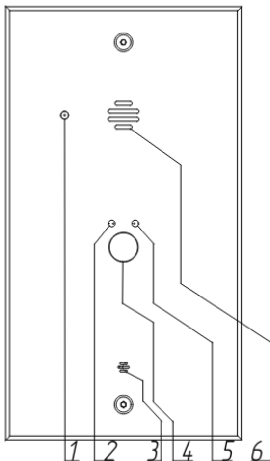
Рисунок 1 - Передняя панель
