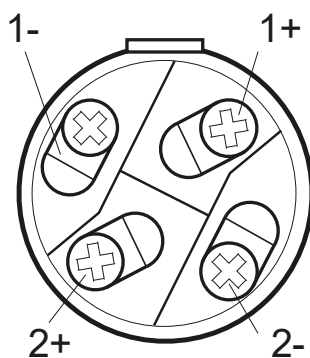
Рисунок 3 – Контакты ответной части разъёма подключения резервного питания.
