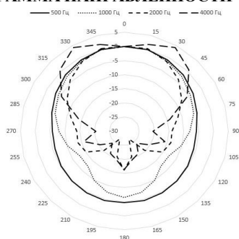
Рис. 2 – Диаграмма направленности оповещателя
