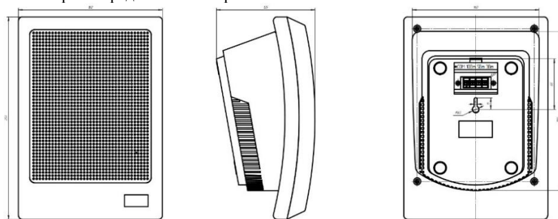
Рис. 1 – Габариты оповещателя
