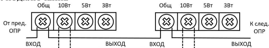
Рис. 3 – Схема подключения оповещателя
