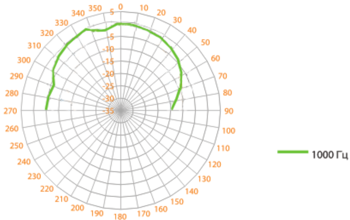
Рисунок 1 – Диаграмма направленности звука оповещателя «Глагол H2-7IP»
