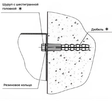
Рисунок 3 - Установка на стену без зацепов
