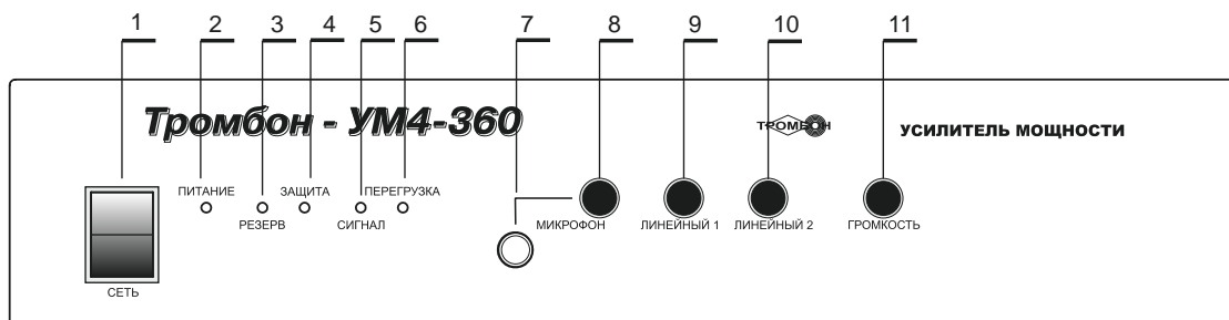
Рис. 1 Эскиз передней панели Усилителя
