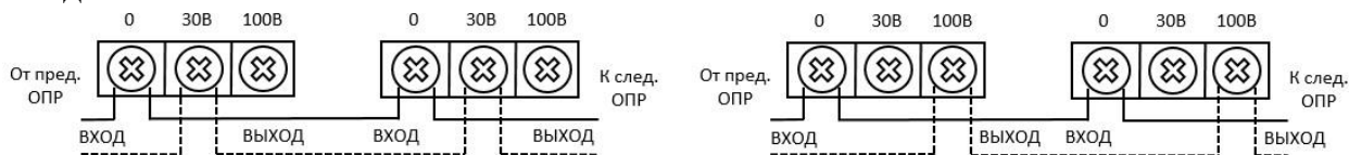
Рис. 3 – Схема подключения оповещателя
