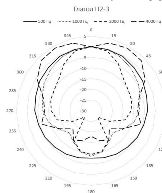
Рис. 2 – Диаграмма направленности оповещателя
