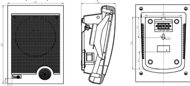
Рис. 1 – Габариты оповещателя
