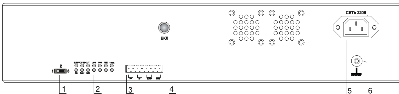
Рис. 2 Эскиз задней панели Коммутатора
