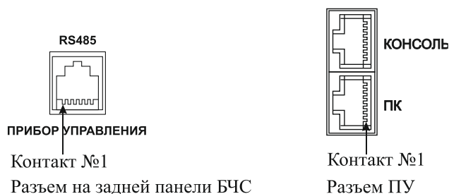
Рис. 3. Схема кабеля для связи «Тромбон БЧС» с прибором управления «Тромбон ПУ-XX».
