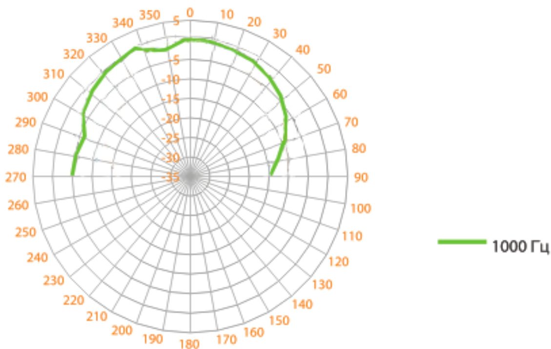
Рисунок 1– Диаграмма направленности звука оповещателя «Глагол НЗ-10IP»
