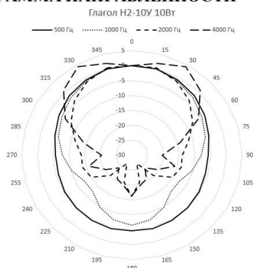
Рис. 2 – Диаграмма направленности оповещателя
