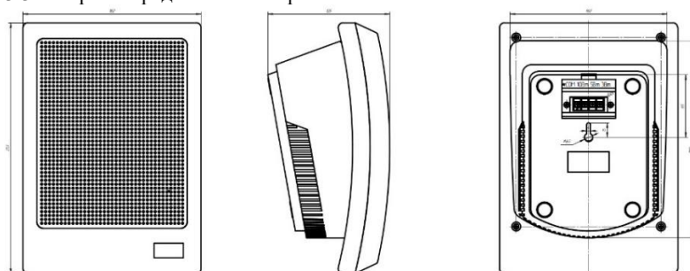
Рис. 1 – Габариты оповещателя
