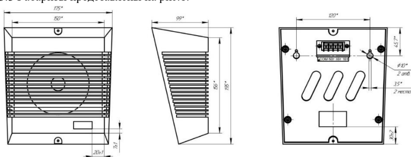
Рис. 1 – Габариты оповещателя
