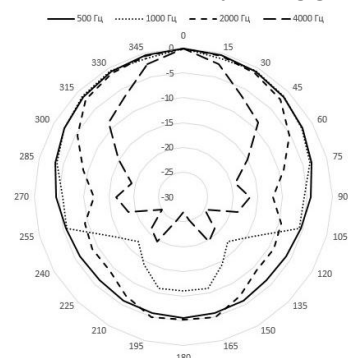
Рис. 2 – Диаграмма направленности оповещателя
