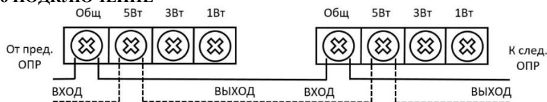
Рис. 3 – Схема подключения оповещателя
