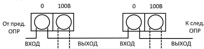
Рис. 3 – Схема подключения оповещателя
