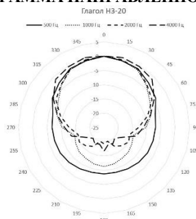
Рис. 2 – Диаграмма направленности оповещателя
