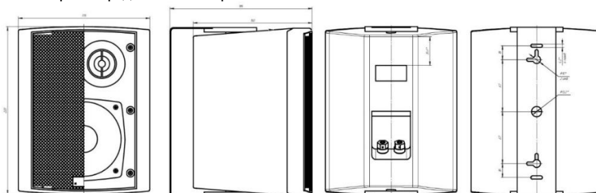
Рис. 1 – Габариты оповещателя
